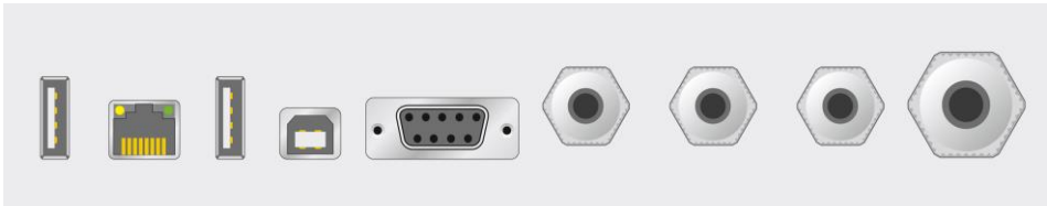
USB1 Host Ethernet USB2 Host USB Device RS232C Kabelverschraubungen für Netzanschluss, M-Bus und I/Os
